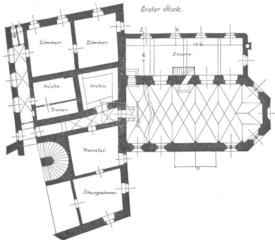
Abb. 8. Grundriß der Kirche und des Benefiziatenhauses, 1936. Maßstab 1:260. (Beschreibung S. 61 und 78.)
