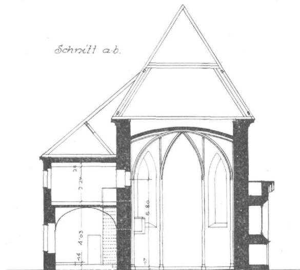
Abb. 11. Schnitt durch die Kirche und den Sakristieanbau. Maßstab 1:260. (Beschreibung Seite 61, 70, 72.)
